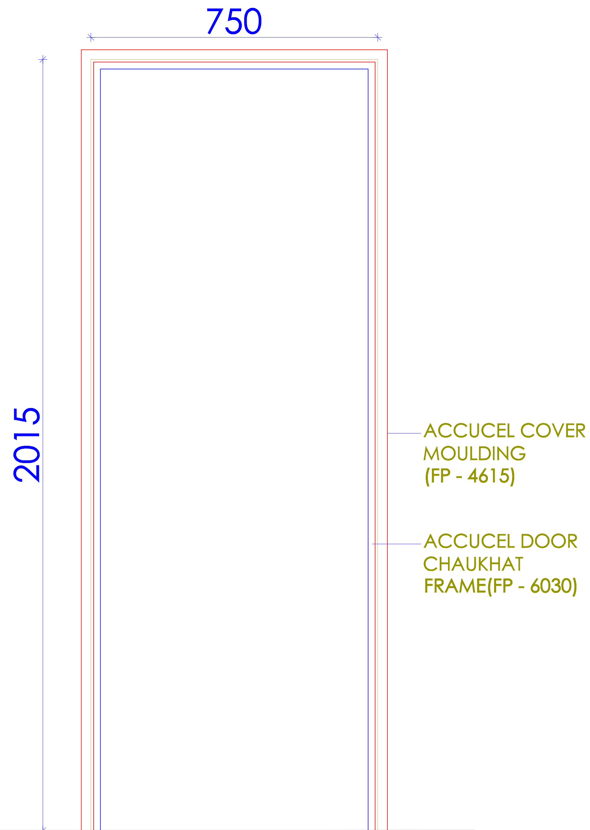
FRAME ELEVATION
